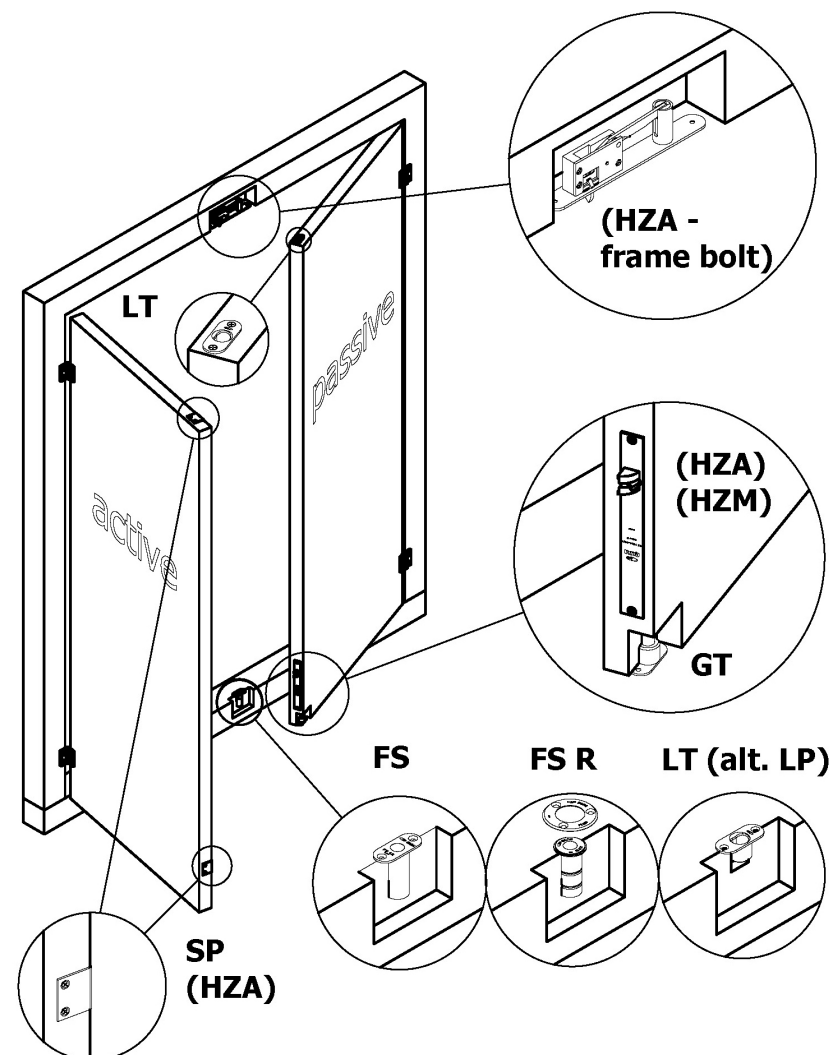
Automatiska karmreglar (HZA-frame bolt), Automatiska kantreglar (HZA) och Manuella kantreglar (HXM)
