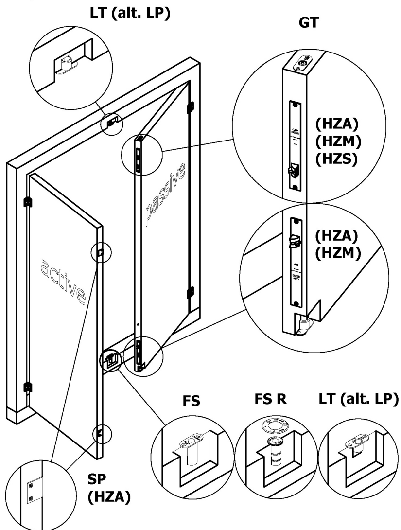
Automatiska kantreglar (HZA), Manuella kantreglar (HXM) och halv-automatiska kantreglar (HXS)
